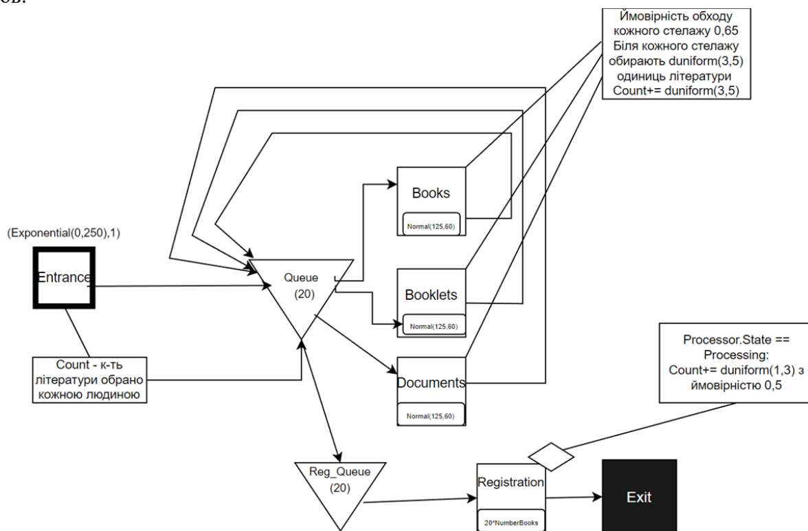
Рисунок 1 – Концептуальна модель імітаційної системи
