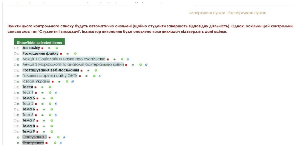
Рисунок 4 – Редагування чек-листу
