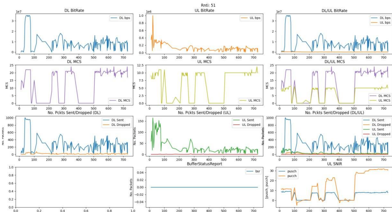
Рис. 2. Графіки трейс-логів для оптимізованої конфігурації
