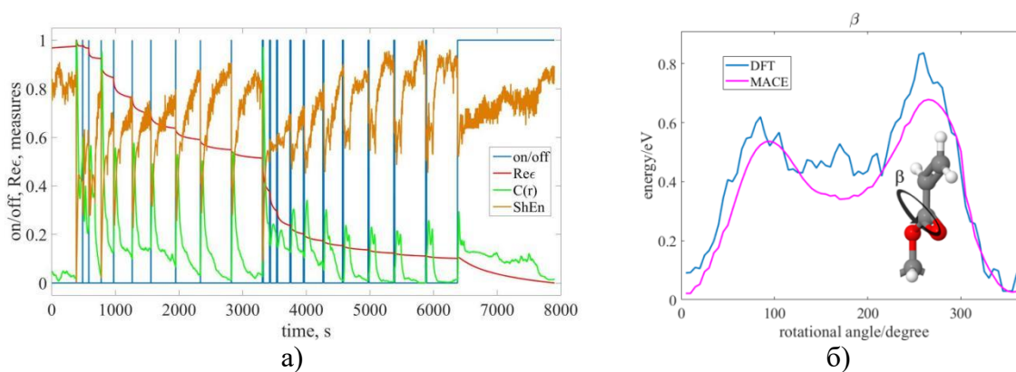
Рис. 2. а) Порівняльна динаміка Re\epsilon , кореляційного інтегралу C(r) та ShEn, розрахована для ковзного вікна тривалістю 250 с з кроком 1 с; б) енергетичний рельєф для \beta релаксації, DFT – розрахунок методом функціоналу електронної густини, MACE – за методикою міжатомних потенціалів машинного навчання.
