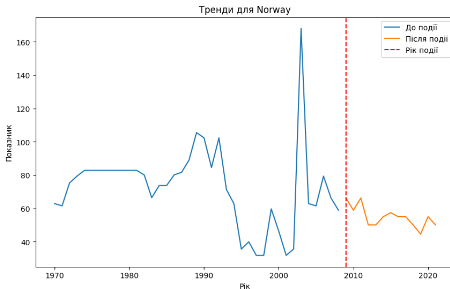
Рис.3 Тренд зміни індексу якості повітря з виділенням екстремуму, що найближчий в ряді після дати введення норми по викиду Євро-5.
