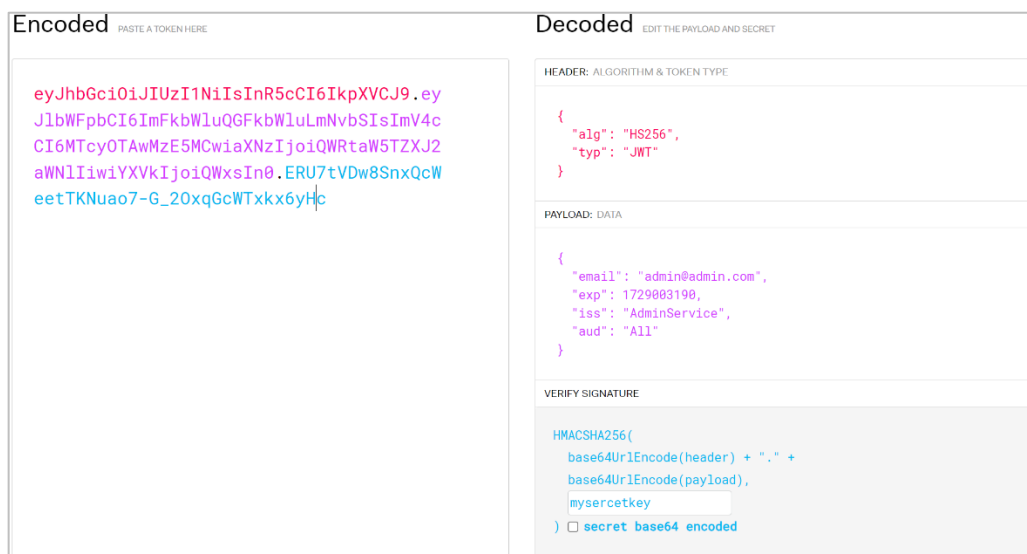
Рисунок 2 - Розшифровка токена на сайті https://jwt.io/
